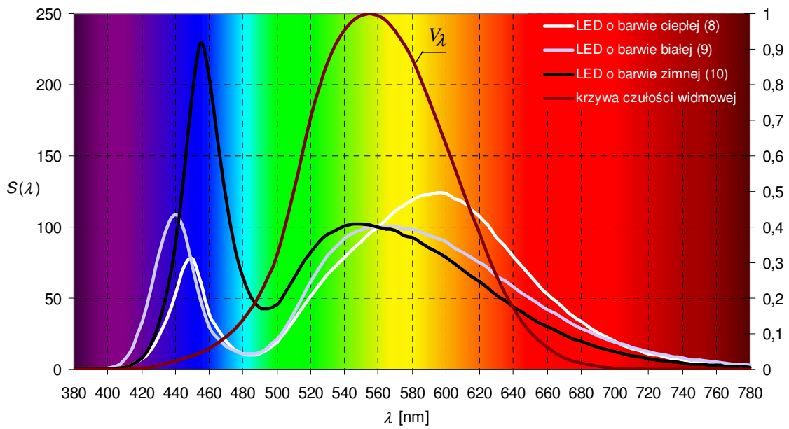
Rys. 6. Krzywe rozkładów widmowych źródeł LED
