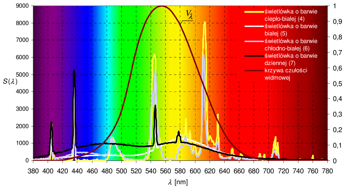
Rys. 5. Krzywe rozkładów widmowych świetlówek liniowych
