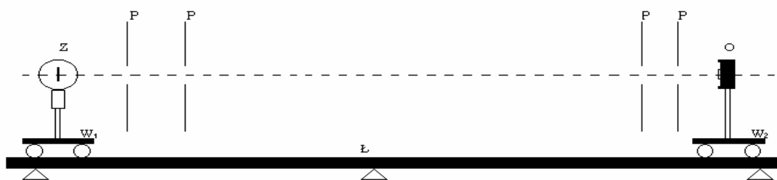
Rys. 1. Schemat stanowiska do wzorcowania luksomierzy:
