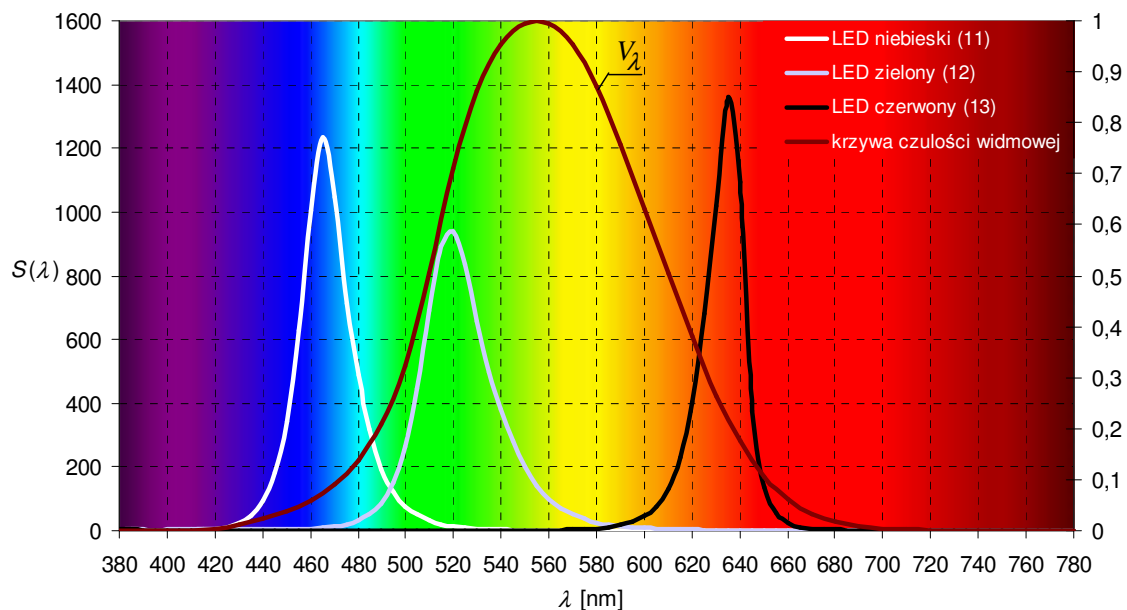
Rys. 7. Krzywe rozkładów widmowych barwnych źródeł LED
