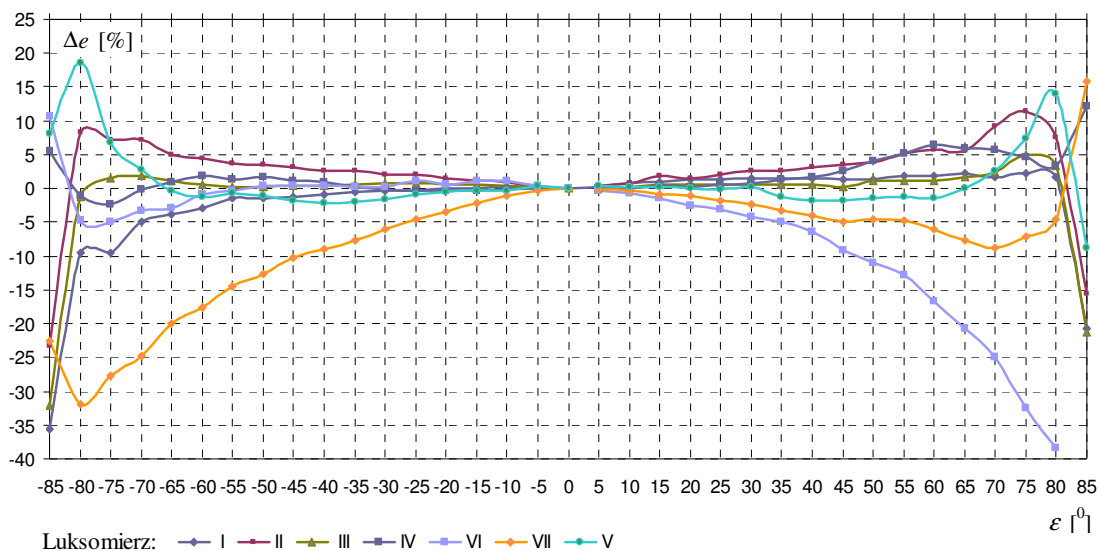
Rys. 3. Błąd kosinusowy luksomierzy
