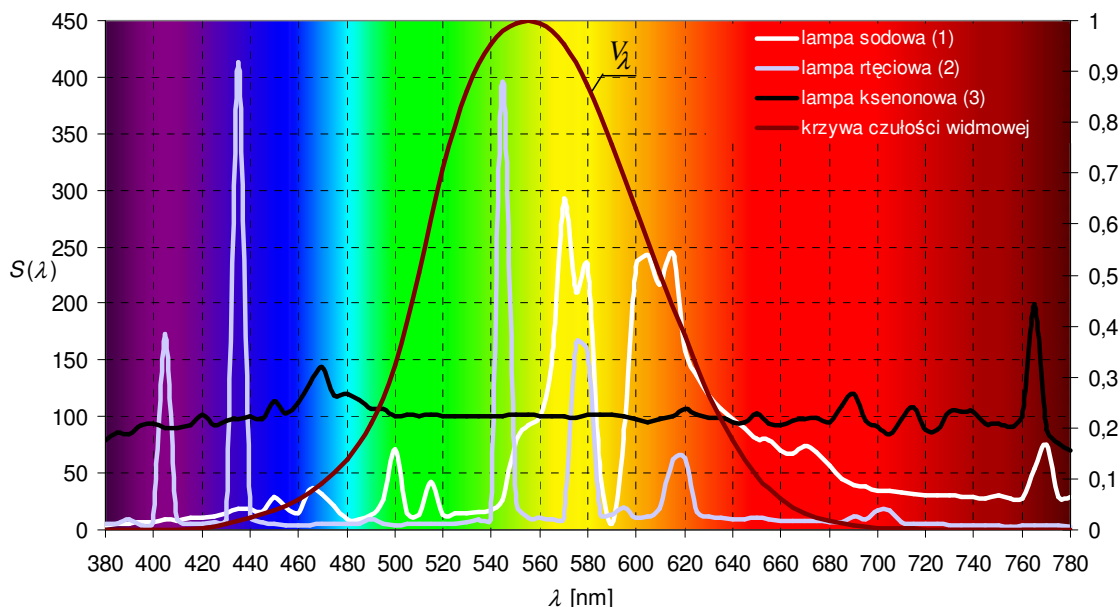
Rys. 4. Krzywe rozkładów widmowych wybranych lamp wyładowczych
