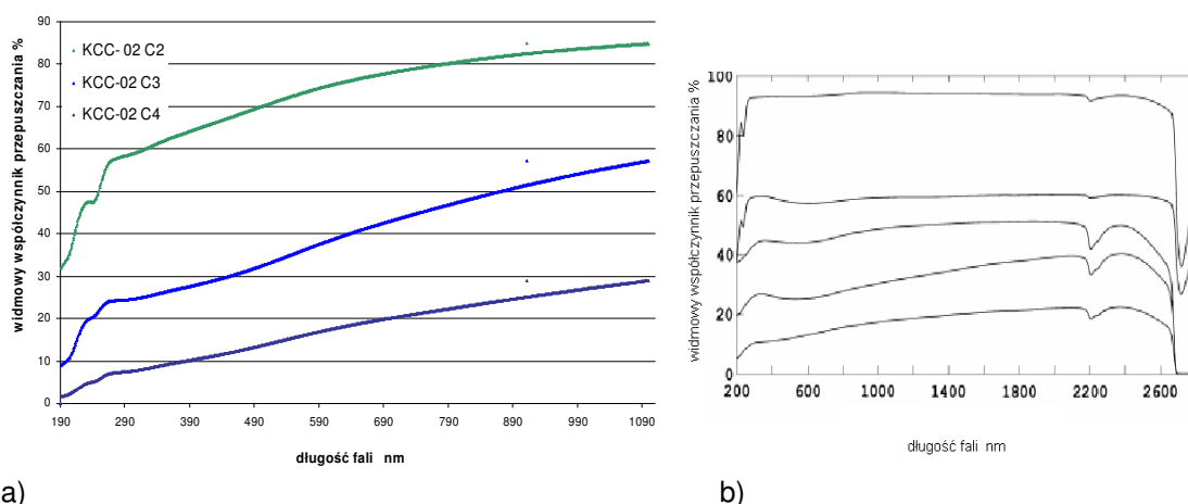
Rys.3. Charakterystyki widmowe filtrów napyłanych
