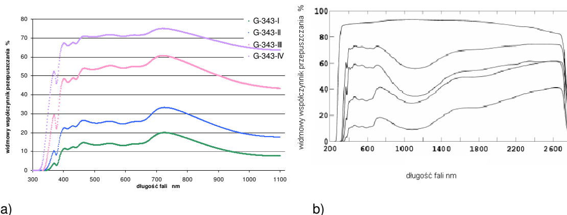
Rys. 2. Charakterystyki widmowe filtrów neutralnych
