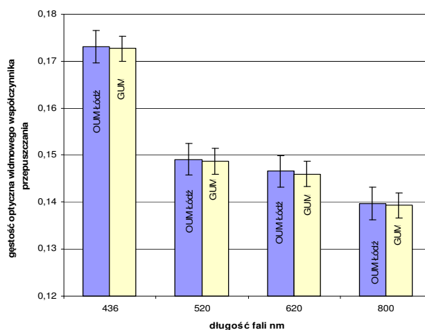
Rys. 6. Gęstość optyczna widmowego współczynnika przepuszczania przy różnych długościach fal dla filtra G-343-IV. Wyniki uzyskane w laboratoriach wzorcujących OUM Łódź oraz GUM
