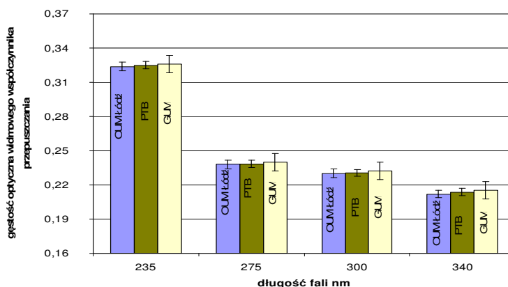
Rys. 8. Gęstość optyczna widmowego współczynnika przepuszczania przy różnych długościach fal dla filtra KCC-02 nr 84 C2. Wyniki uzyskane w laboratoriach wzorcujących OUM Łódź, PTB oraz GUM
