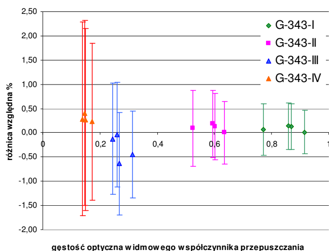
Rys. 7. Różnica względna pomiaru gęstości optycznej widmowego współczynnika przepuszczania pomiędzy laboratorium OUM Łódź oraz GUM
